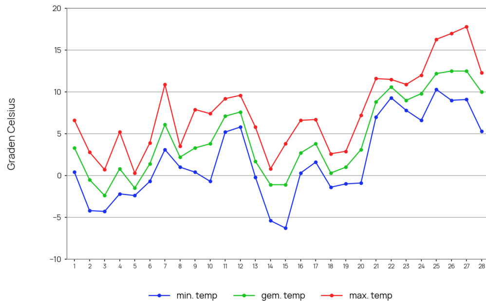
Temperatuurverloop Meteo Almelo, februari 2026
