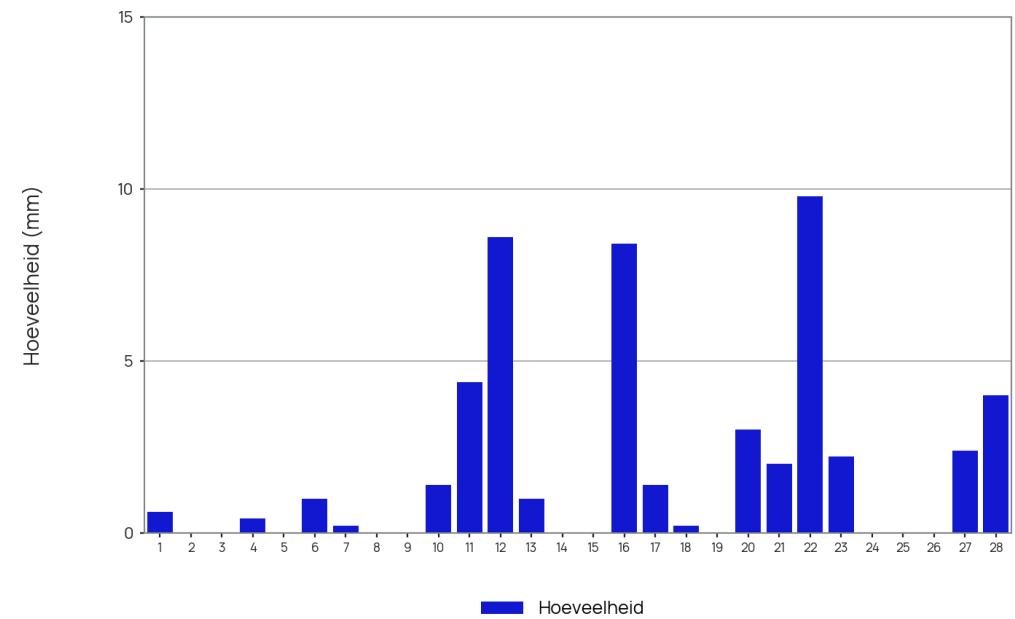
Neerslag Meteo Almelo, februari 2026
